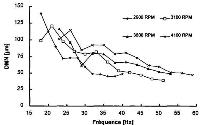
Fig. 6. DMN en fonction de la fréquence. Satellites. Q = 8 \text{ mL/min} .
