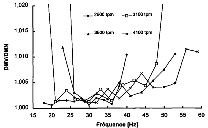
Fig. 5. DMV/DMN en fonction de la fréquence. Gouttes primaires. Q = 8 \text{ mL/min} .
