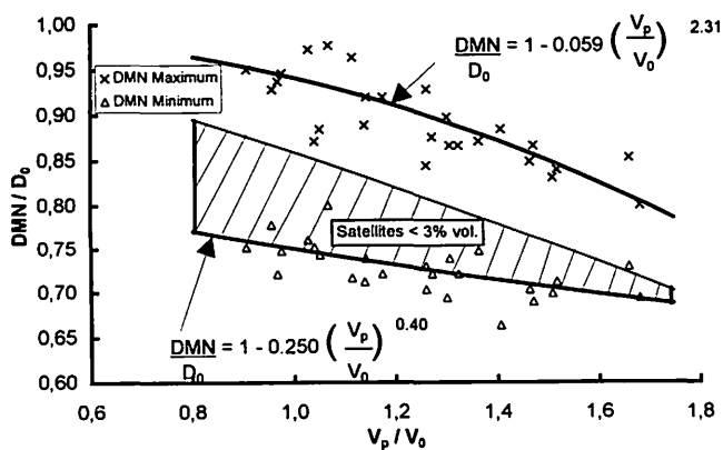
Fig. 8. Évolution du DMN/D_0 en fonction du ratio V_p/V_0 . Zone hachurée: moins de 3% vol. en satellites.
