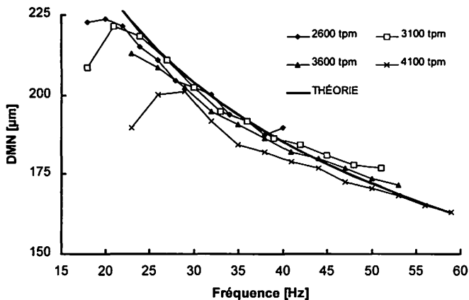
Fig. 4. DMN en fonction de la fréquence. Gouttes primaires. Q = 8 \text{ mL/min} .
